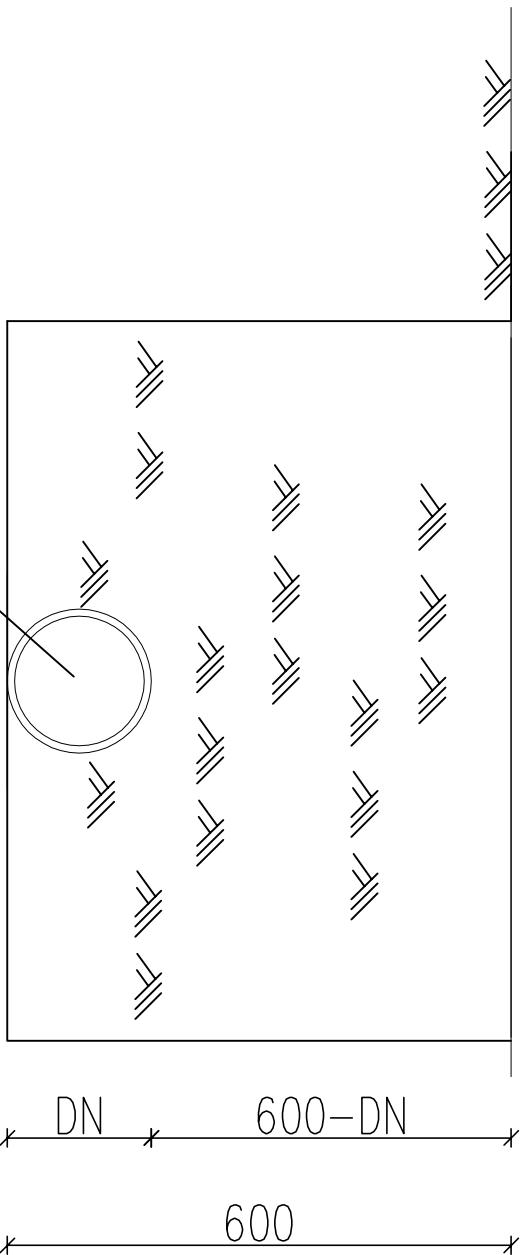
1.25MPa压力DN32PE管 断面图(1:100)
