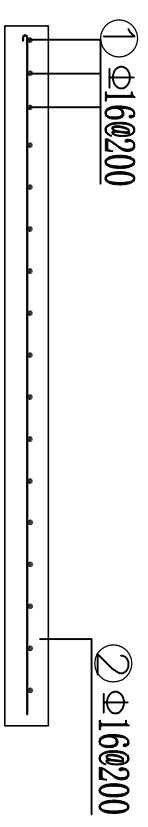
现浇底板配筋图 1:50
