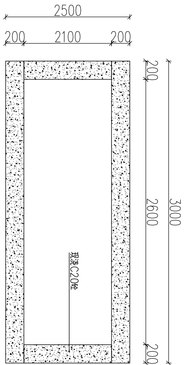
蓄水池平面图 1:20
